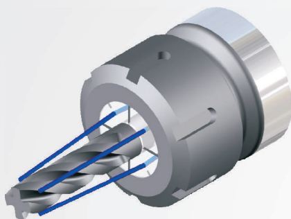
Abb.: Spannanzge mit »Cool Tool«-Bohrungen für Werkzeuge ohne Innenkühlung
