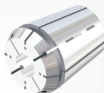
Abb.: Spannanzge mit »Cool Tool«-Bohrungen für Werkzeuge ohne Innenkühlung
