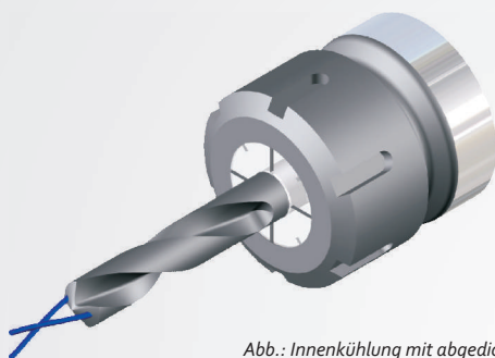
Abb.: Innenkühlung mit abgedichteter Spannanzge
